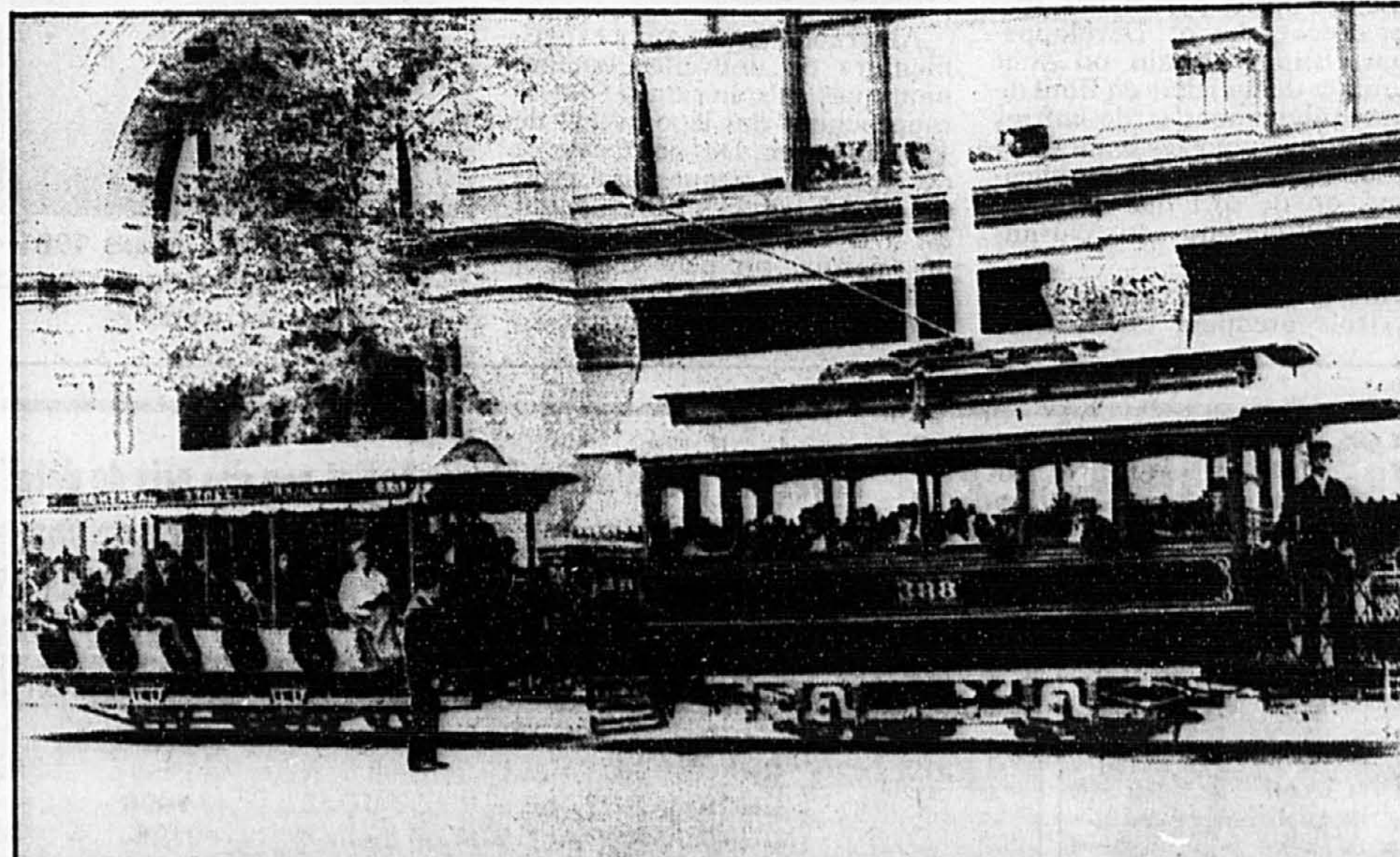
Ce tramway électrique, photographié devant le magasin Morgan en 1894, remorque un vieux tramway à traction animale que l'on utilisera jusqu'en 1897 afin de pouvoir accueillir plus d'usagers.
