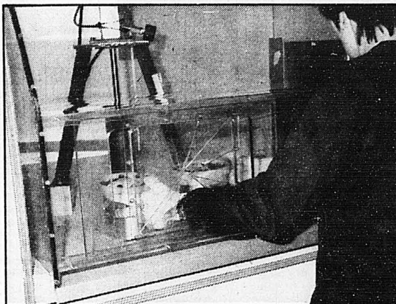
Poste de travail pour la fabrication des bombes sphériques, derrière un écran de sécurité.
