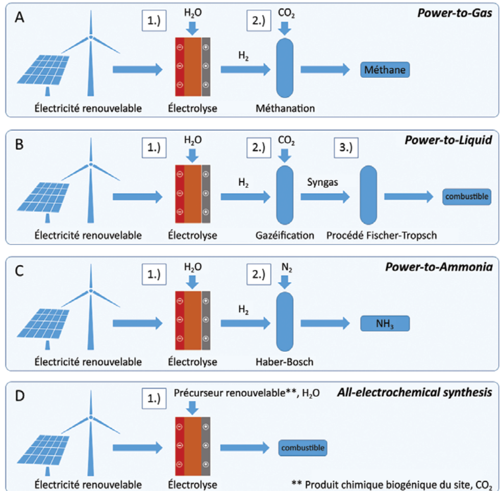
Figure 3 : Possibilités de conversion du Power-to-X © 2018 Energies [4].
