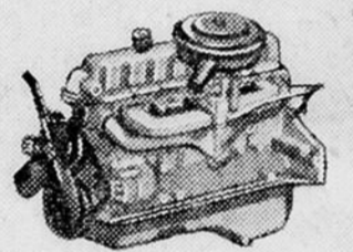
Moteur 6 cylindres Astro-Six de 230 po. cu., développant 140 CV.
