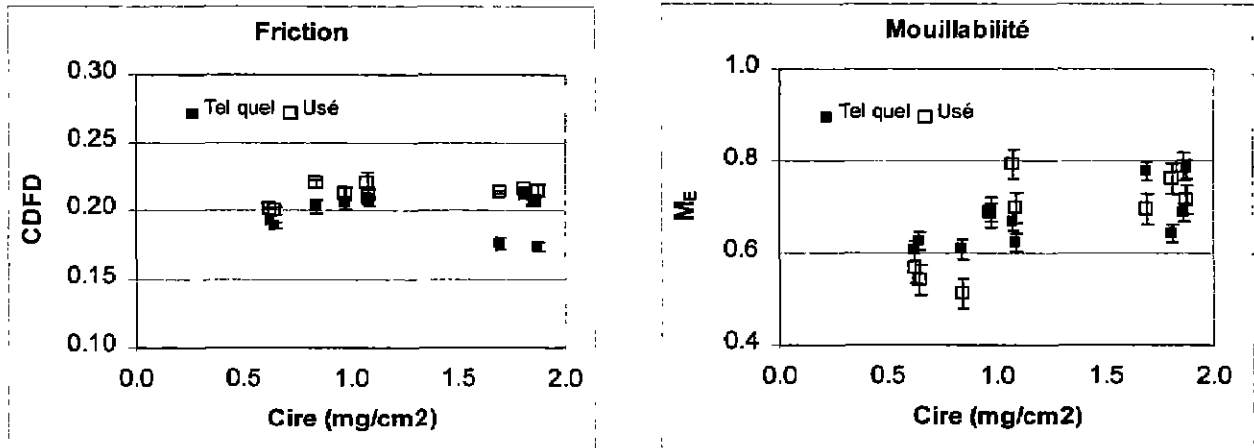
Figure 12 Impact de la quantité de cire sur la friction d'un revêtement de vinyle. Surface cirée telle quelle et usée mécaniquement
