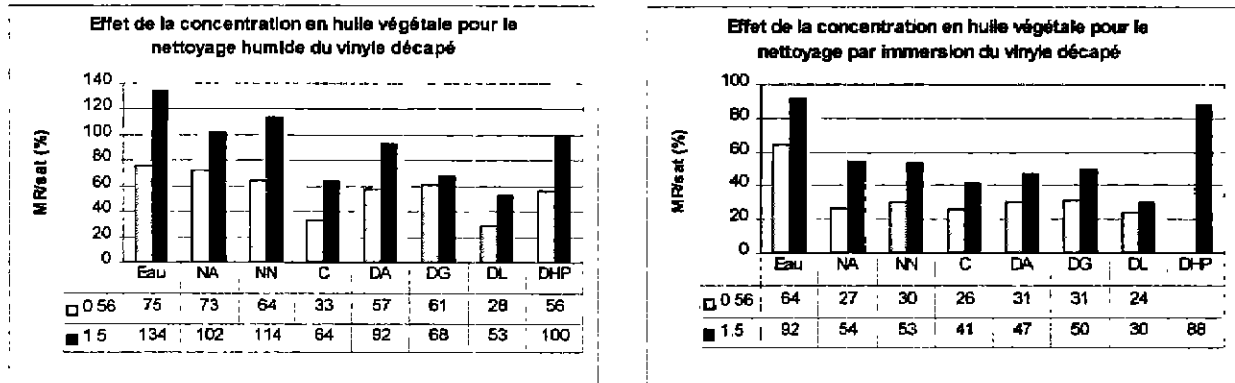
Figure 36 Matière résiduelle (MR/sat) suite à un nettoyage humide (gauche) ou par immersion (droite) du vinyle décapé selon la concentration (mg/cm 2 ) d'huile végétale à 23 °C
