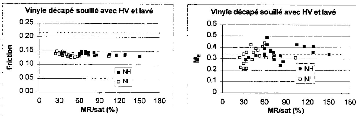
Figure 39 Évolution du CDFD (Friction) et de la mouillabilité par l'eau ( M_E ) selon la concentration résiduelle en huile végétale sur le vinyle décapé suite à un nettoyage humide (NH) ou par immersion (NI) à 23 °C. Les pointillés correspondent aux conditions propres.
