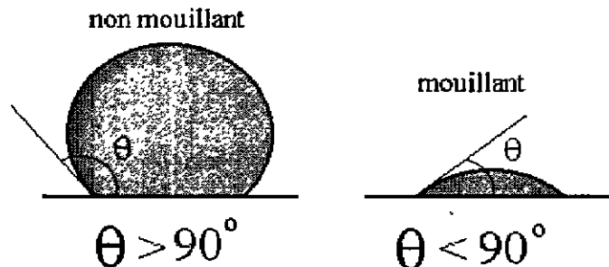
Figure 3 Illustration de conditions mouillante et non mouillante pour une goutte sur une surface
