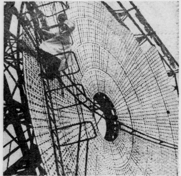
ENERGIE SOLAIRE : Le miroir géant du Laboratoire d'énergie solaire de Mont-Louis, en France, qui a près de 10 mètres de diamètre et se compose de plus de 3,500 morceaux de verre. Ce miroir parabolique, en concentrant les radiations sur l'orifice d'un four solaire, permet d'y créer une température de 3,000 degrés C. Les recherches entreprises dans le but de capter la chaleur solaire sont de la plus haute importance pour l'avenir des régions arides pauvres en énergie. (Photo Laboratoire d'énergie solaire, Mont-Louis)
