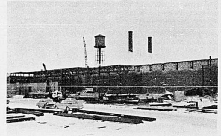
Photo prise à la Cie de Papier Rolland, où on a confié à la firme Omega, la construction de la bâtisse devant abriter la nouvelle machine No 8.
