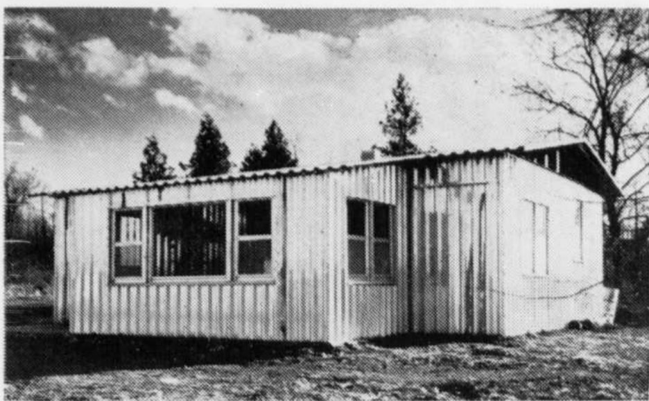
LE FUTUR CAMP DE CHASSE ET DE PECHE, avec sa cuisine, ses deux chambres à coucher et son living room qui pourrait être contenu dans une boîte de trois pieds de largeur, douze pieds de longueur et sept pouces de profondeur. Fait d'aluminium, il répondra au désir de nombreux sportifs. La Cie Kingston Frameless House, espère fabriquer bientôt de ces camps pour le marché canadien.
