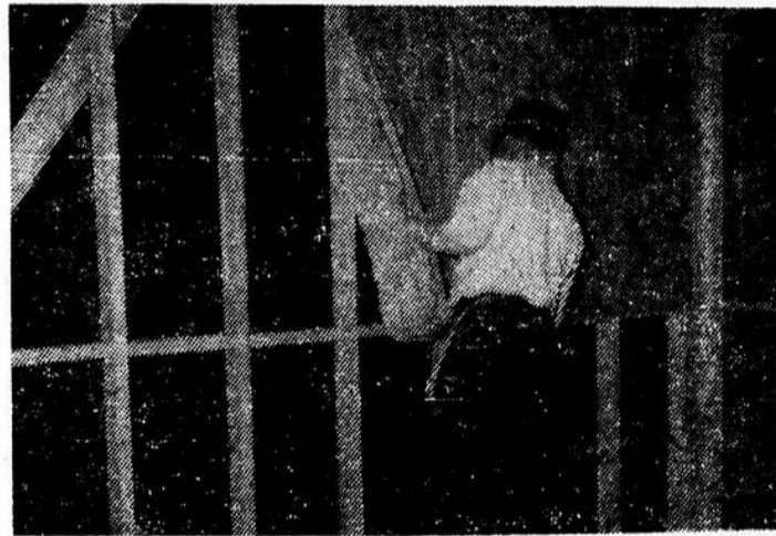
Dans les murs, 3" de laine minérale en natte.
