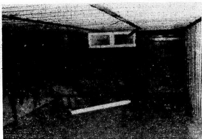
Pose du polyéthylène avant de couler le plancher en béton du sous-sol.
