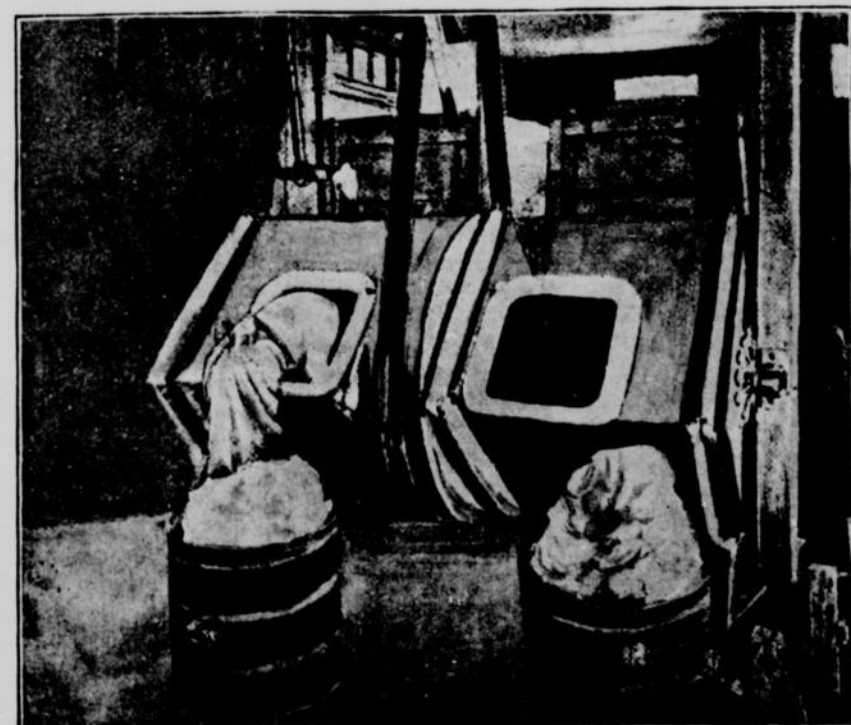
Baratte à vapeur contenant 350 gallons de crème
