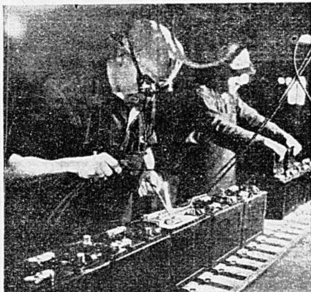
Des masques filtrent la poussière de plomb en flottement dans l'air pendant le couplage des plaques par séries.
