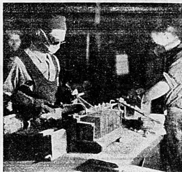
Au montage: L'ouvrier de droite remplit les batteries d'acide sulfurique et l'autre effectue le raccordement des cellules.
