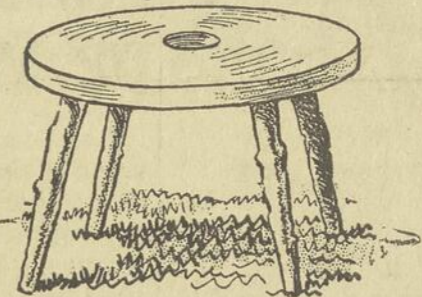
MÉTAMORPHOSE D'UNE MEULE FAITES UNE CHARPENTE CARRÉE AVEC DU PIN DE 1" OU DES RONDINS DE CÈDRE POUR Y FIXER DES PIEDS RUSTIQUES OU DE SIMPLES RONDINS DÉGROSSIS. HAUTEUR APPROX.: 16" DU SOL.
