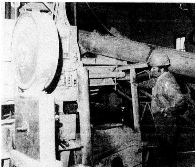
L'employé ci-dessus, M. Maurice Lemelin de St-Raphaël, vérifie la qualité du mélange de gravier et de ciment en vrac et s'assure ainsi du poids et de la teneur en humidité de ce ciment qui est destiné à la fabrication des blocs en béton. Il s'agit d'une des premières opérations sur la chaîne de production.
