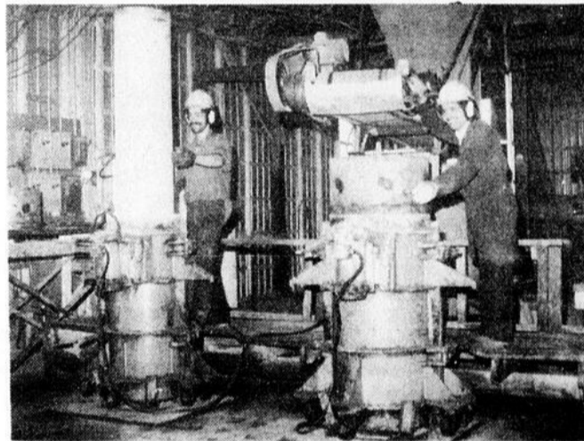
Les deux employés Daniel Grenier et Jacques Asselin s'affairent au démoulage des tuyaux qui sont fabriqués par le principe de la vibration. Ce nouvel agrandissement de l'usine a nécessité des investissements de plus de $100,000.
