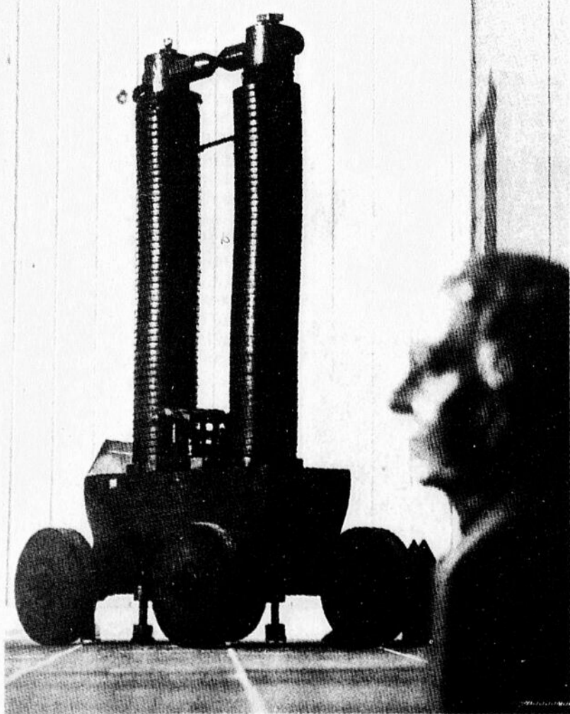
Le grand électro-aimant de H. C. Orsted, de 1846. Au premier plan, le buste de Orsted façonné en aluminium.
