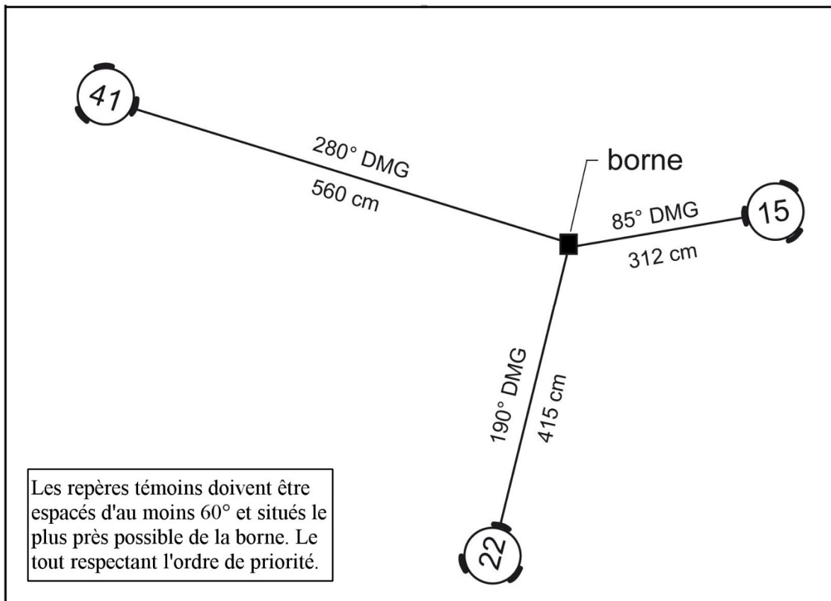
Figure 6 Alignement des marques des repères témoins par rapport à la borne
