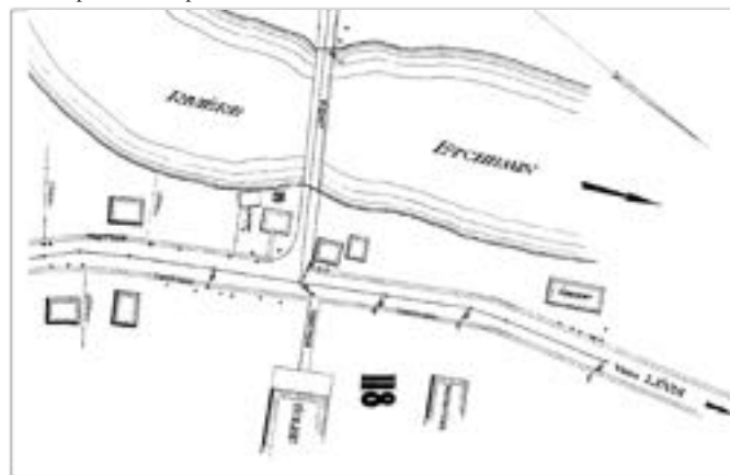
Plan montrant le lot cadastral No 118 dans le Village de St-Henri, comté de Lévis avant la construction du nouveau pont sur la rivière Etchemin, 13 août 1936
