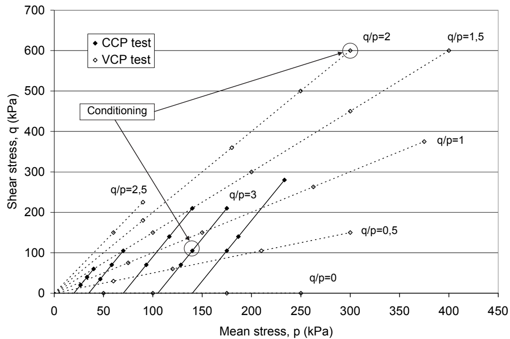
Figure 7 États de contraintes appliqués lors du conditionnement des éprouvettes et des essais triaxiaux avec confinement constant (CCP) ou variable (VCP) (Doucet, 2006)
