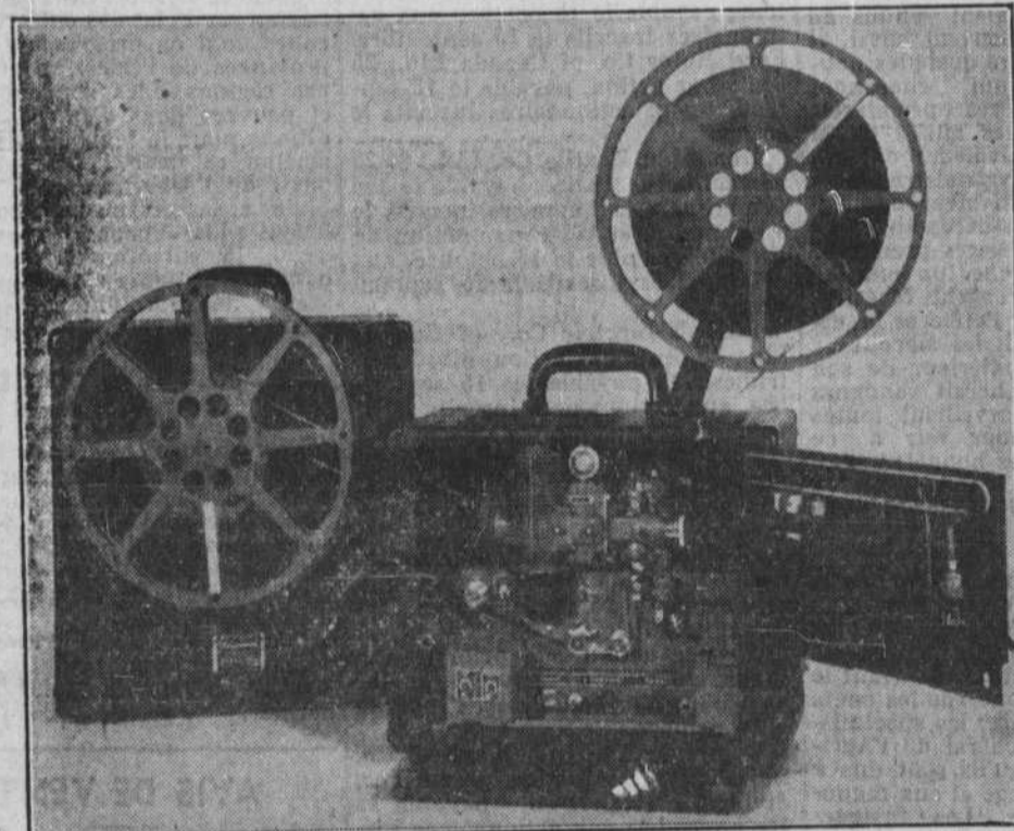
LE PROJECTEUR EN FONCTIONNEMENT... TOUS LES BOUTONS DE CONTRÔLE SONT ACCESSIBLES LA PETITE PORTE INFÉRIEURE PEUT AUSSI ÊTRE REFERMÉE.
