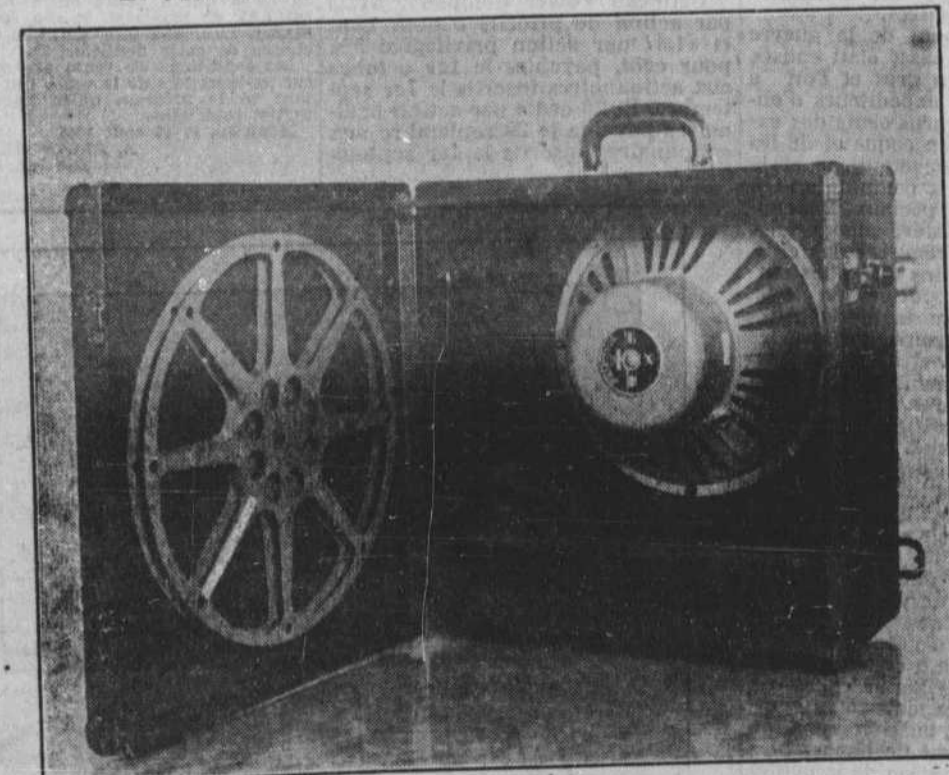
LE HAUT-PARLEUR DU MODELE "156" SPECIAL 12" DE DIAMÈTRE A AIMANT PERMANENT MUNI DE 50 PIEDS DE CABLE — CAISSE LUXEUSE ET PRATIQUE
