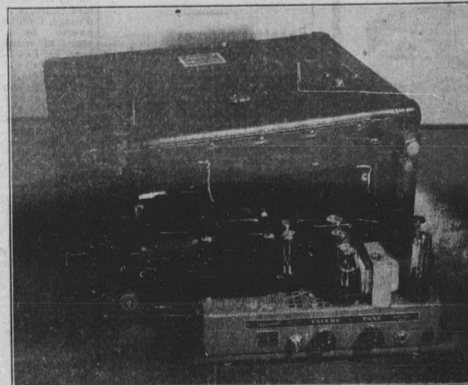
L'AMPLIFICATEUR EST ENTIÈREMENT DÉTACHÉ PERMETTANT UN REMPLACEMENT RAPIDE DES LAMPES, ET PLUS FACILE LA VÉRIFICATION DU CIRCUIT DE L'AMPLIFICATEUR.
