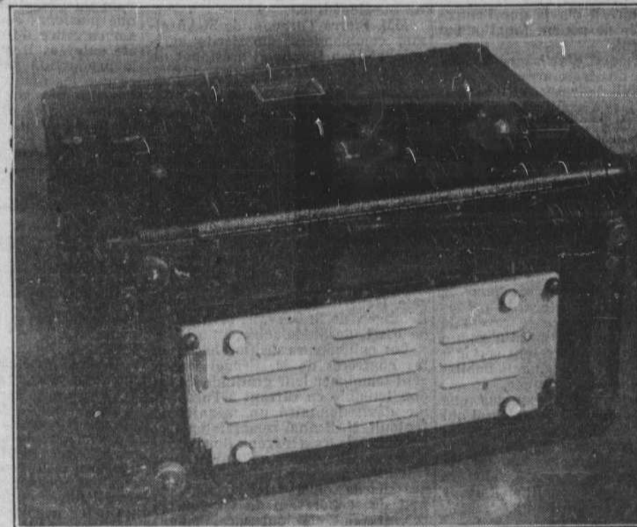
AMPLIFICATEUR DANS LA BASE... DEMONTABLE RAPIDEMENT SANS DÉFAIRE L'APPAREIL QUATRE GROSSES VIS MOLLETÉES LE SOUTIENNENT EN PLACE.
