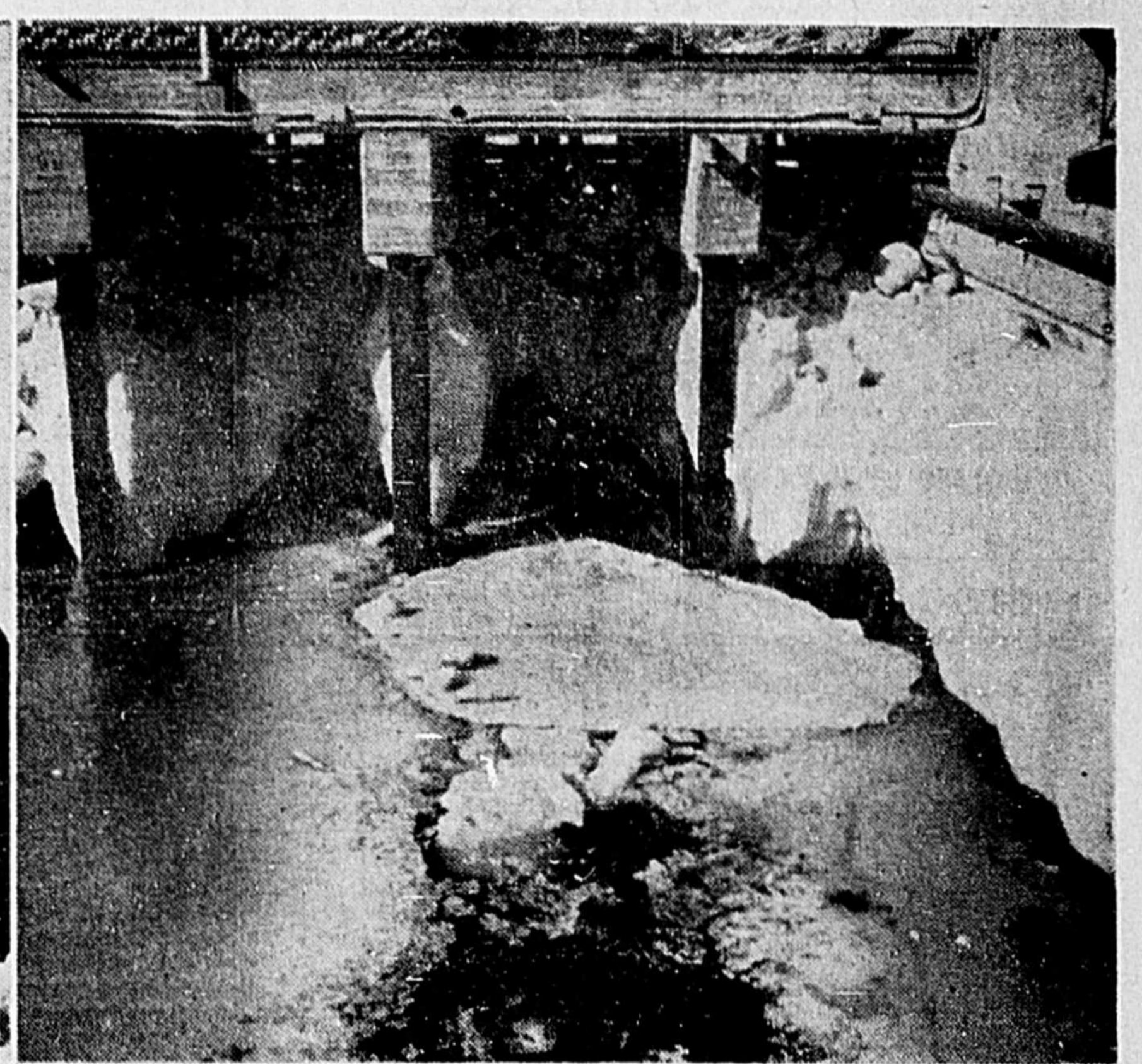
Cette photo illustrant le dessous des quais de Saguenay Terminals nous fait voir les arcades creusées dans la glace par les molécules d'eau déplacées par des bulles d'air comprimé. Au premier plan, on peut voir le bouillonnement des bulles faisant des trous de 8 pieds de diamètre dans la glace. Le tuyau de polyéthylène repose à 40 pieds de la surface. (Photo-scoop)
