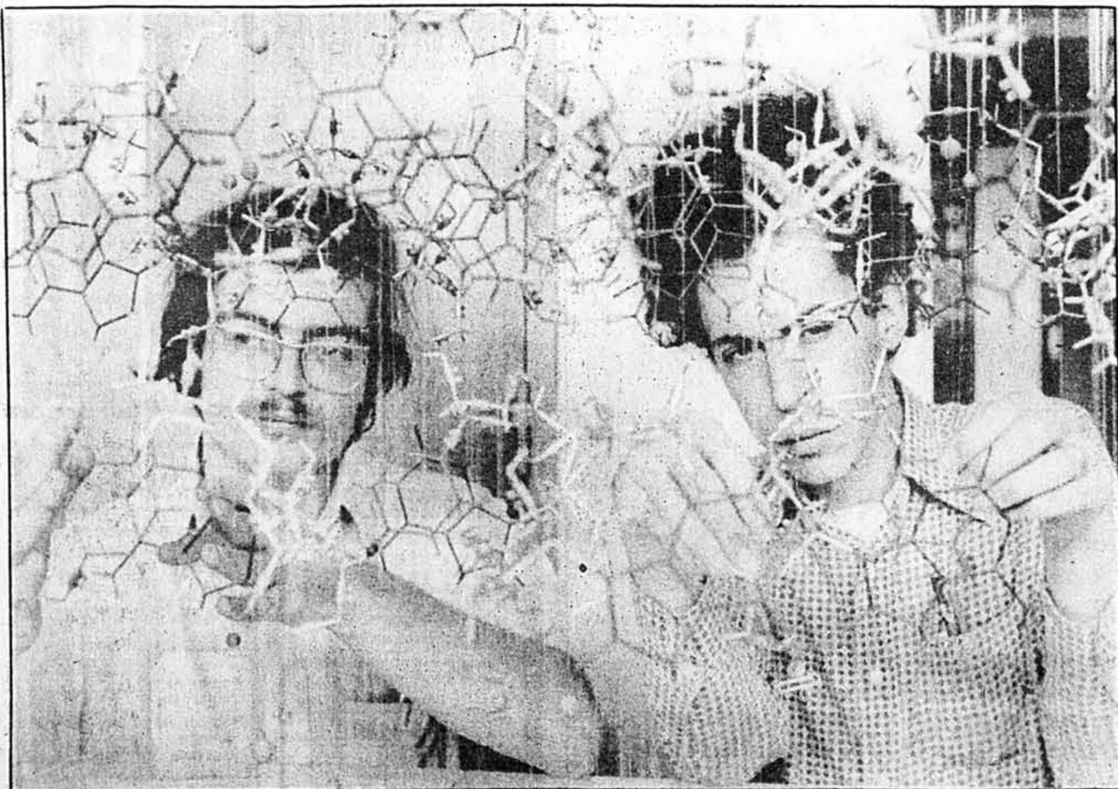
L'ADN est une substance appartenant au groupe des protéides. Elle est isolée par extraction du noyau cellulaire. La molécule, très complexe, est constituée par deux spires enroulées en sens inverse
