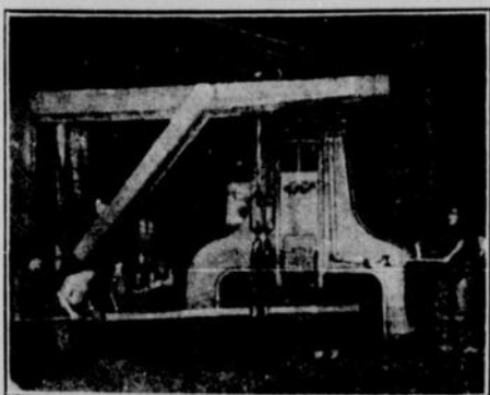
Forgeage d'une bielle de locomotive
