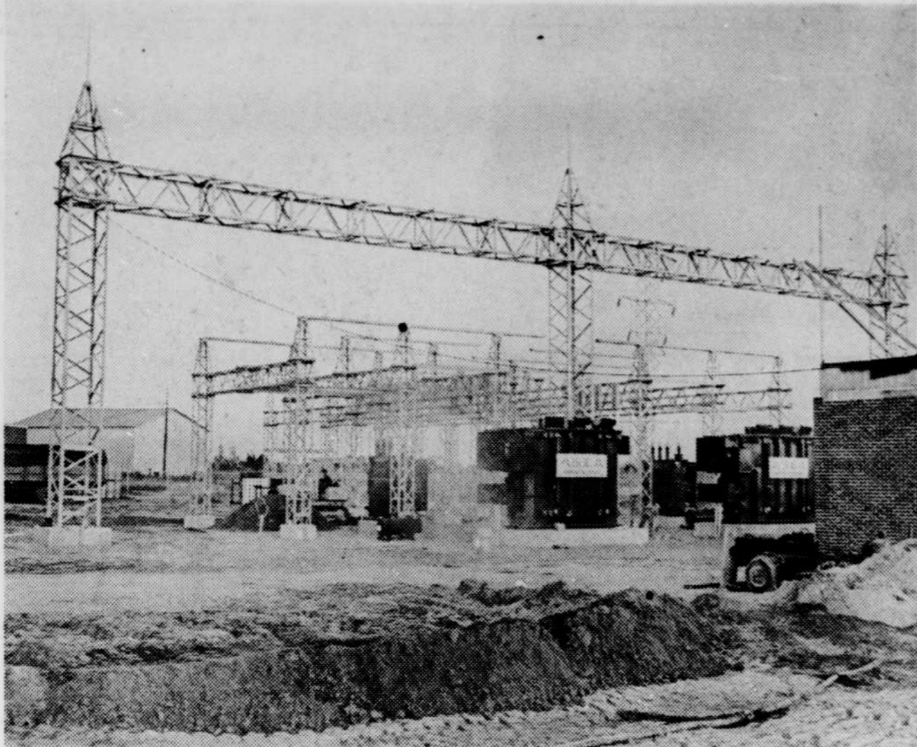
Environ 35 pour cent des travaux de construction du nouveau poste de distribution Bois-Francs à Victoriaville, sont complétés. Ce nouveau poste doit être en service dès octobre prochain. (Cliché Le Nouvelliste)
