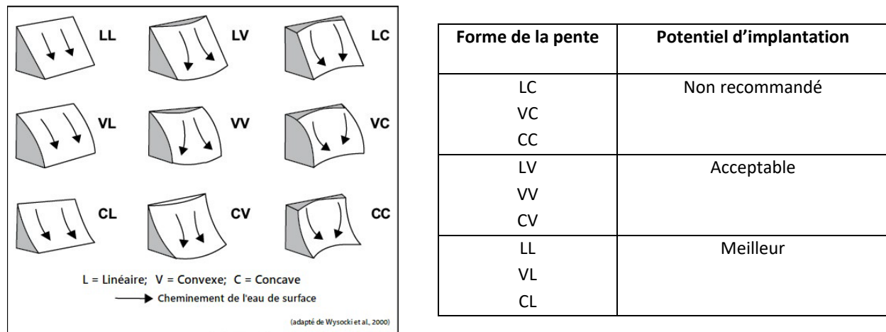
Figure 3.10 : Représentation des formes de pente du terrain (source : SSDS, 2017) et potentiel d'implantation d'un OEIS selon l'USEPA
