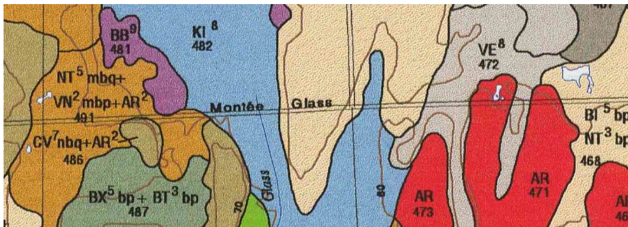
Figure 3.6 : Extrait de la carte pédologique du comté de Saint-Jean (source : Lamontagne et coll., 2001, AAC – Contient de l'information visée par la Licence du gouvernement ouvert - Canada )
