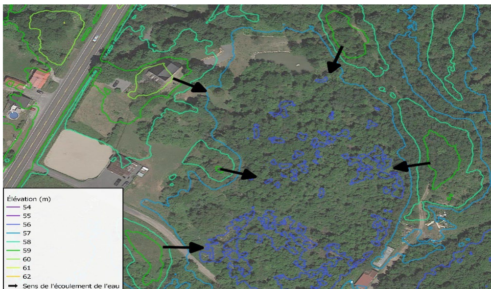
Figure 3.5 : Relevé topographique provenant des données LiDAR
