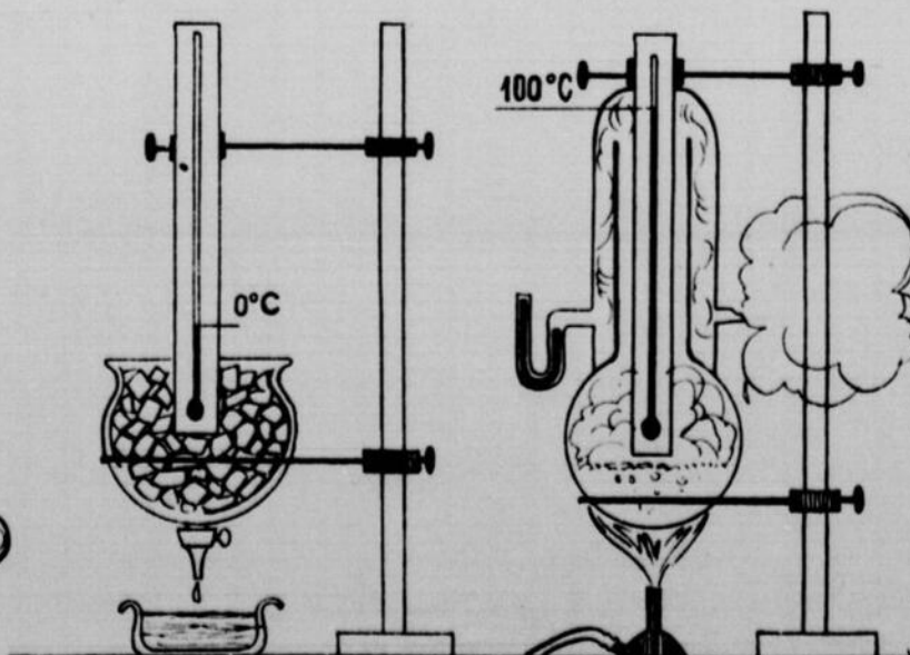
OBTENTION DU POINT DE GLACE FONDANTE
