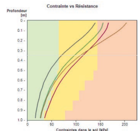
Figure 3 : Effets sur le profil de sol
