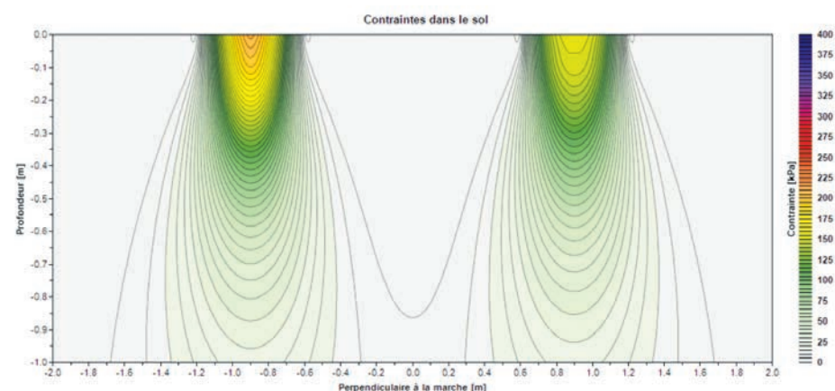
Figure 5 : Contraintes dans le sol
