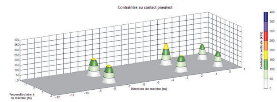
Figure 4 : Pression sur le sol à la surface
