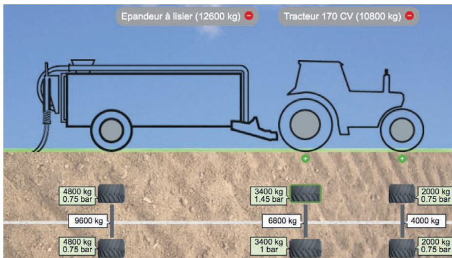
Figure 1 : Configuration de la machinerie
