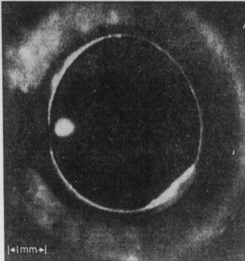
La "goutte" électrique est représentée par le point brillant, à gauche. Quant au grand anneau blanc, c'est le reflet de la lumière infrarouge émanant des bords du cristal de germanium. La goutte mesure 1-30e de pouce de diamètre et contient, selon les chercheurs, quelque dix mille milliards de charges électriques.
