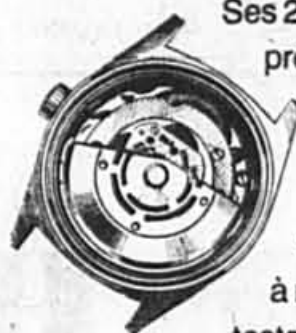
Le mécanisme à rotor Rolex Perpetual
