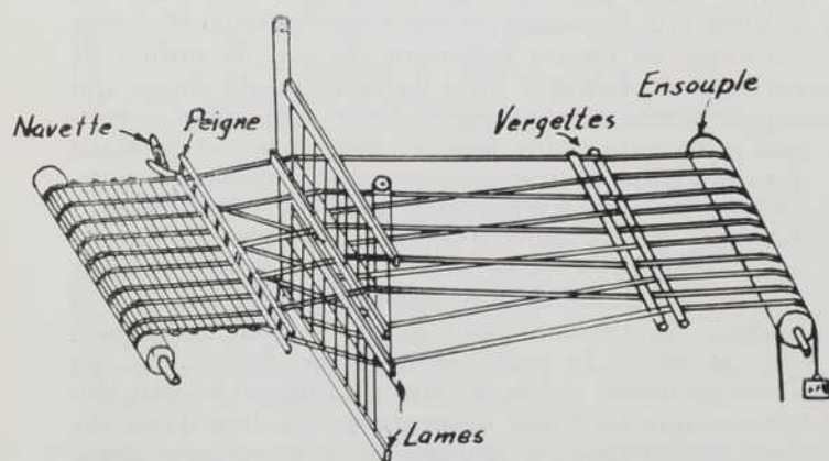
Fig. 1 — Schéma d'un métier à tisser. La navette va et vient successivement au travers de la pièce tissée.
