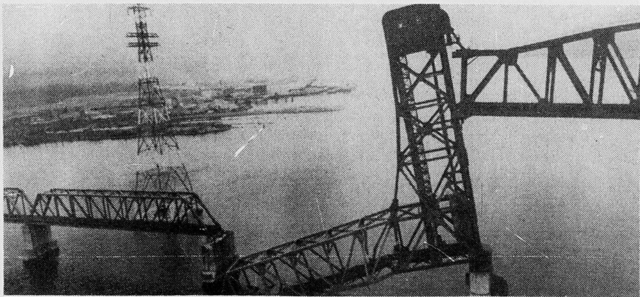
KNOCK OUT — Le pont de chemin de fer du Canadien National enjambant la partie nord du port de Vancouver s'est effondré hier après qu'il eut été heurté par un cargo
