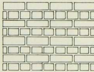
carreaux et boutisses
