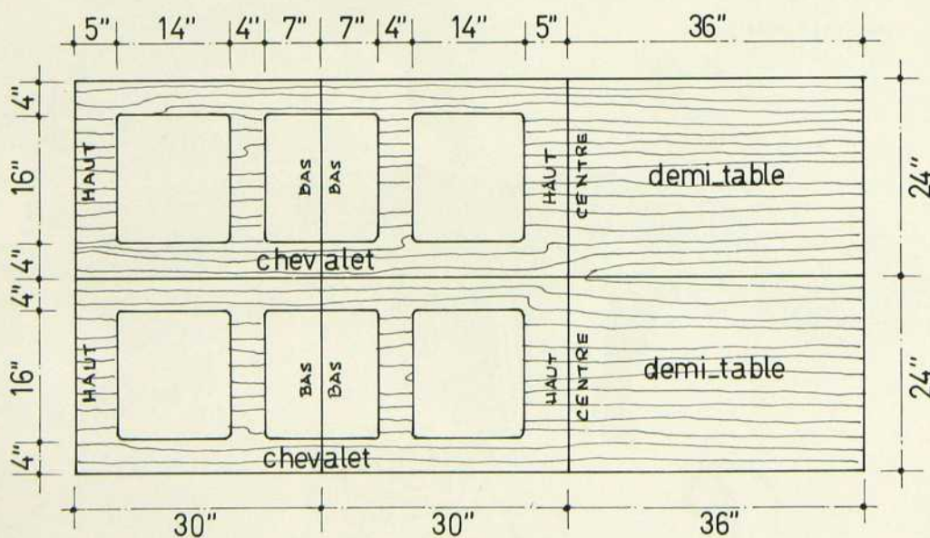
① PLAN DE COUPE DU PANNEAU DE 4' x 8'
