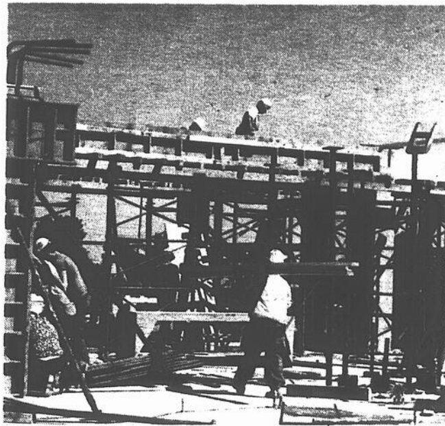
On a commencé, toujours à l'extrémité nord, à couler les dalles de béton qui relient entre eux les piliers, donnant ainsi naissance au plancher du troisième étage.
