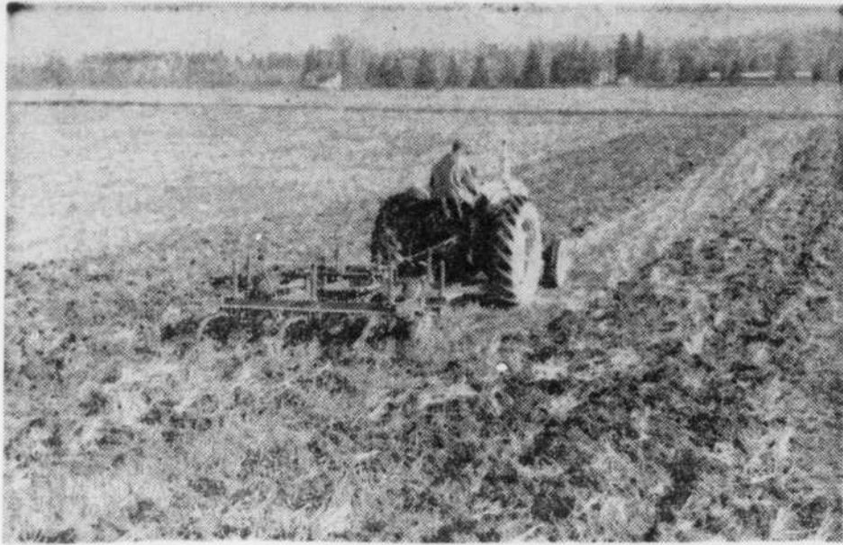
La charrue Graham, un genre de cultivateur servant à bouleverser et à détruire le gazon. Ce travail se fait généralement à l'automne. Au printemps, on pratique les autres façons culturales afin de mettre le sol en état de recevoir la semence.
