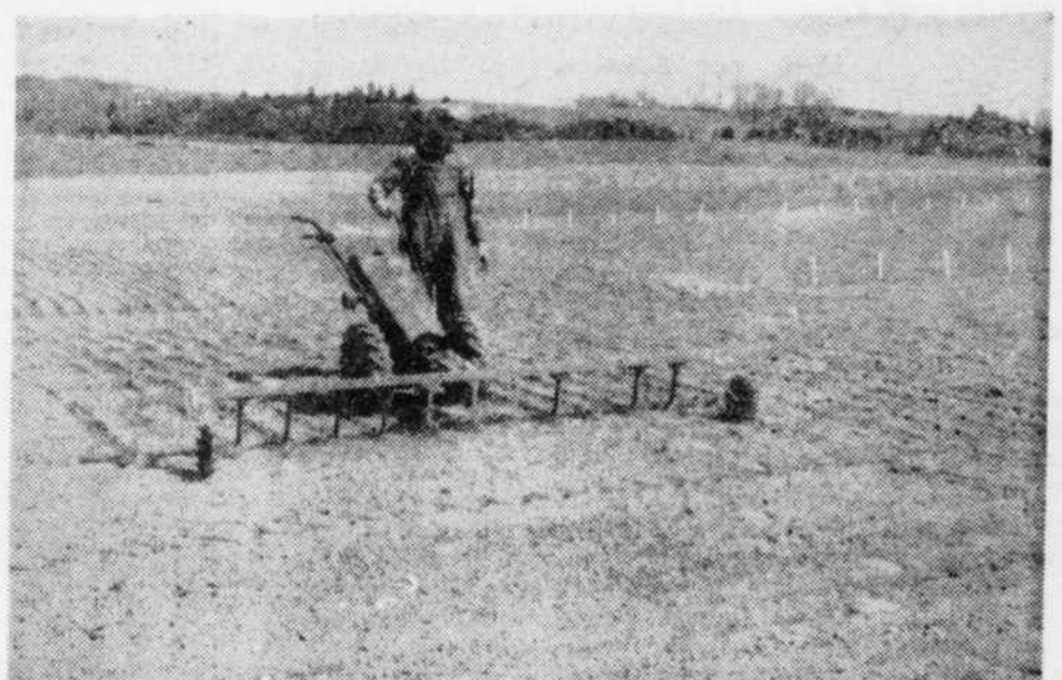
Ensemencement des essais de variétés de céréales au moyen d'un semoir expérimental. Chaque parcelle à céréales comprend quatre rangs de 18½ pieds de longueur. On sème une seule parcelle à la fois et la semence est pesée pour chacune d'elles.
