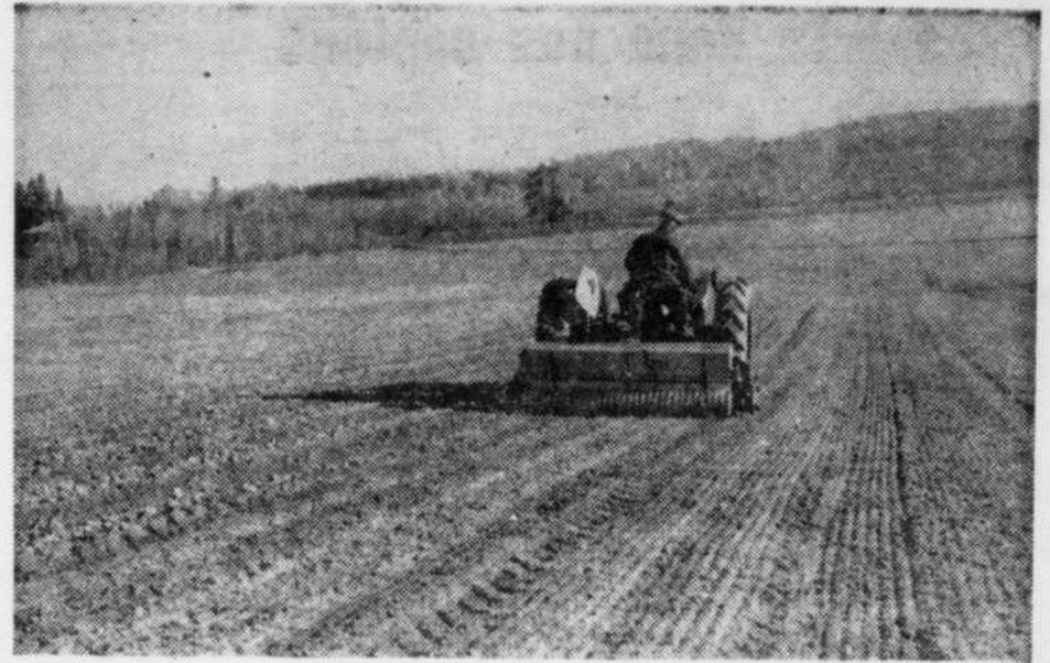
Le semoir Brillion sert surtout à l'ensemencement des graines de plantes fourragères. Une fois la céréale enssemencée, ce genre de semoir raffermi le sol. La machine peut aussi servir de rouleau capable de préparer le terrain pour l'ensemencement des parcelles.
