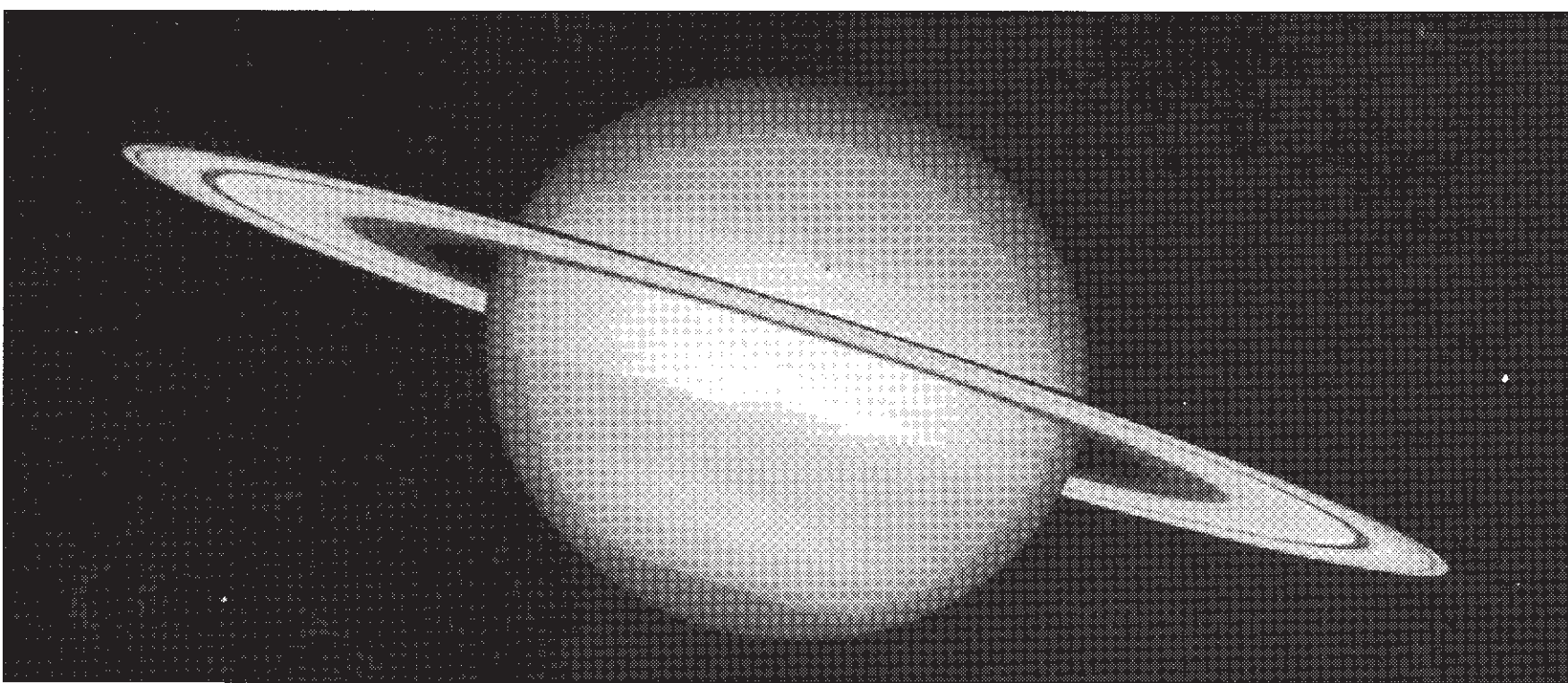
Invisibles sur cette photo de Saturne prise par le télescope spatiale Hubble, en 1998, les nouveaux satellites s'ajoutent aux 18 déjà répertoriés. Ils sont de petite taille et ont des orbites irrégulières qui peuvent être regroupées en plusieurs familles.
