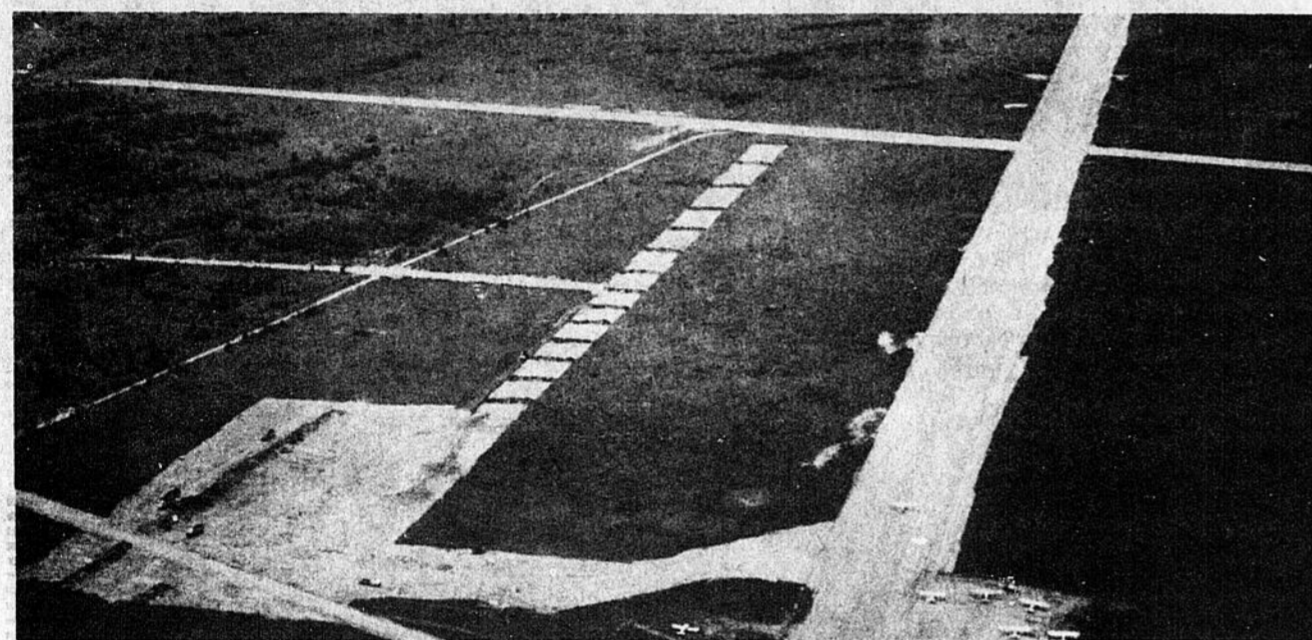
AEROPORT — Pour l'aéroport de St-Méthode, les bénévoles ont fait un bon travail. Ainsi, ont-ils prêté de leur équipement mécanique pour améliorer la piste existante, en l'élargissant de 100 à 150 pieds, ainsi que pour faire une sortie et un stationnement d'avions.
