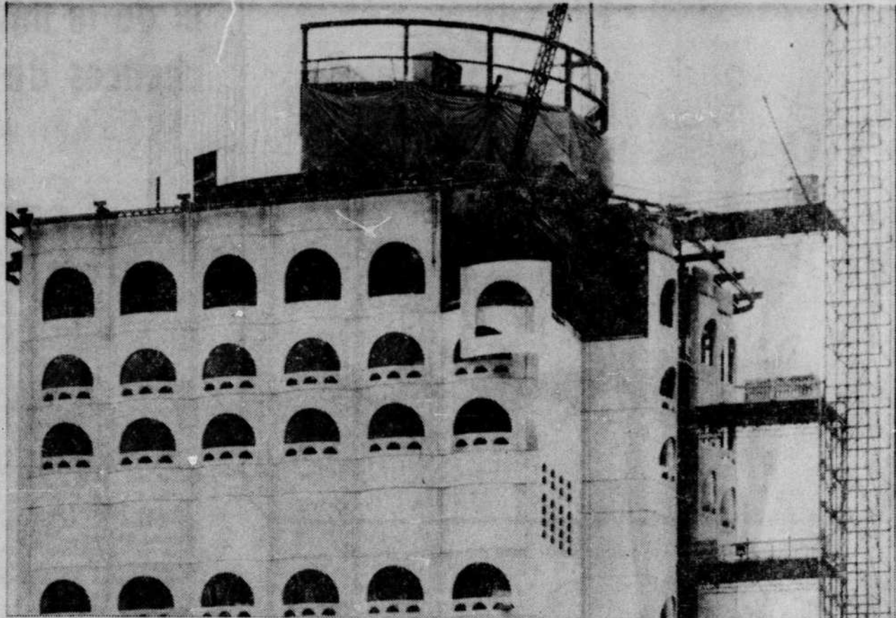
Les travaux de construction du Château Champlain ont franchi une étape importante ces jours derniers avec l'installation du dernier panneau de revêtement en béton précontraint. Cette manœuvre, accomplie à l'aide d'une grue installée au faite de l'édifice, avait débuté en juillet. Les travaux de finition d'intérieur se poursuivront maintenant à l'abri des intempéries. L'ouverture de l'hôtel du Canadien Pacifique, qui s'intègre dans l'ensemble des immeubles de la Place du Canada, doit avoir lieu au début de 1967.
