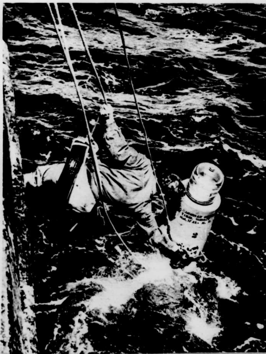
Dans les eaux du golfe Saint-Laurent, le North Star VI vient de repérer sur l'eau, grâce à sa couleur rouge, un courantographe ramené à la surface.
