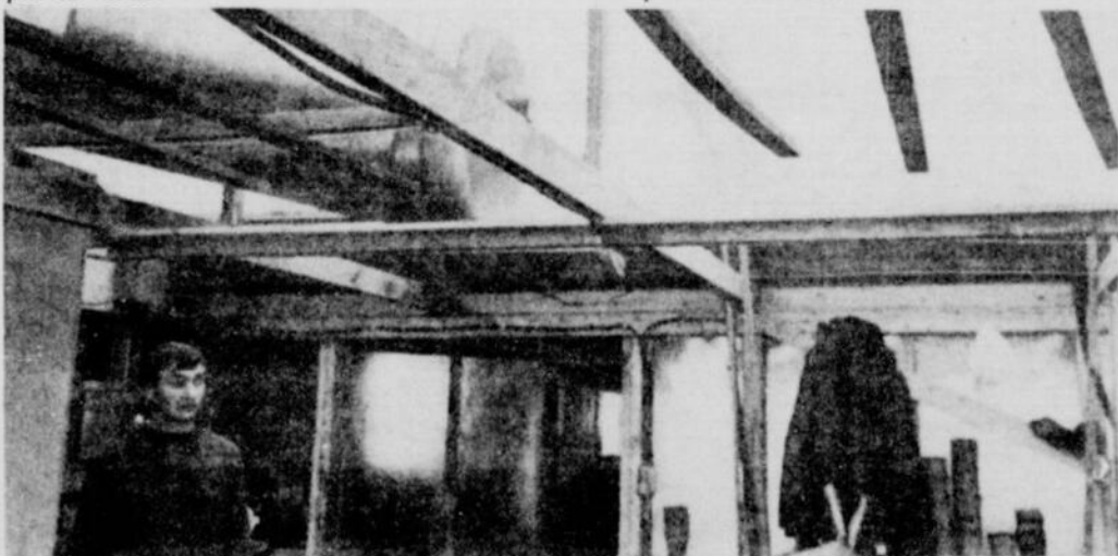
M. Bélisle a imaginé de faire circuler de l'air entre les deux couches de polyéthylène grâce à des ventilateurs. En haut, à gauche, le tuyau qui amène l'air.
