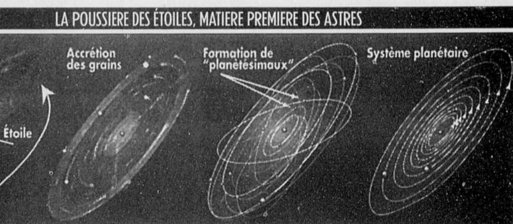
Certaines étoiles sont entourées d'un disque de matière en rotation formé de gaz et de particules. Ces grains de matière s'agrègent progressivement entre eux sous l'effet des forces gravitationnelles. Ils forment alors de petits corps de quelques kilomètres, les planétésimaux, qui, à leur tour, serviront de matière à la formation des planètes. Ce processus s'étend sur plusieurs dizaines de millions d'années.
