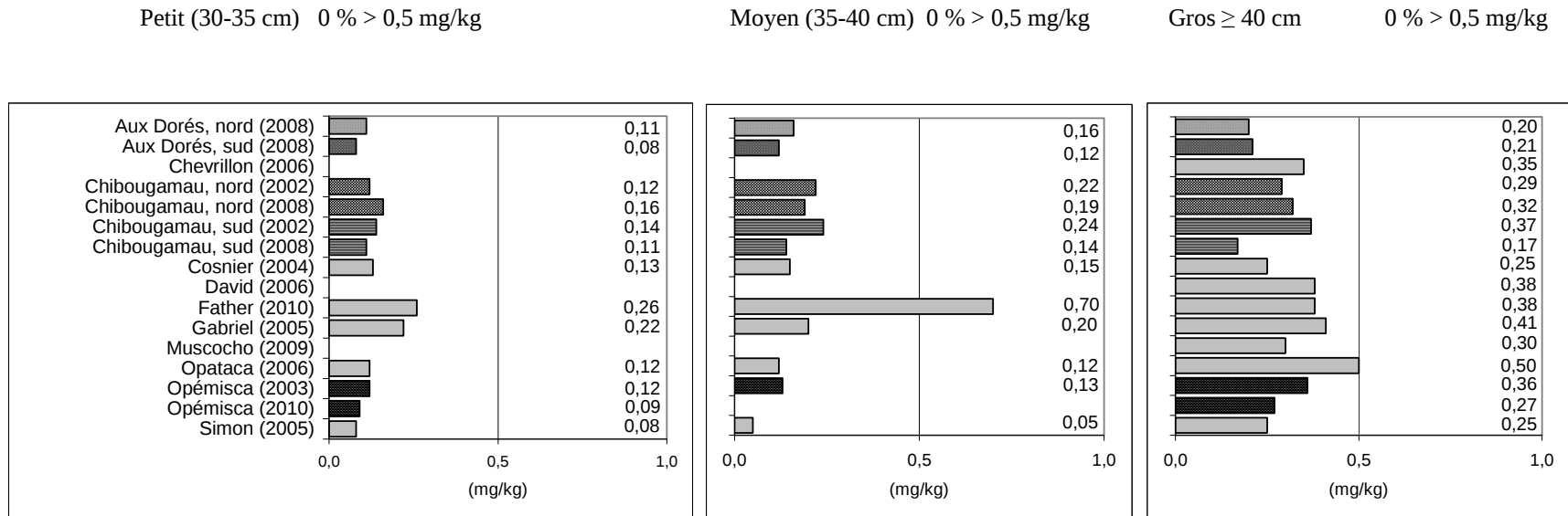
Figure 9 Teneurs en mercure dans la chair du meunier rouge des lacs de la région de Chibougamau et d'Oujé-Bougoumou (2002-2010)
