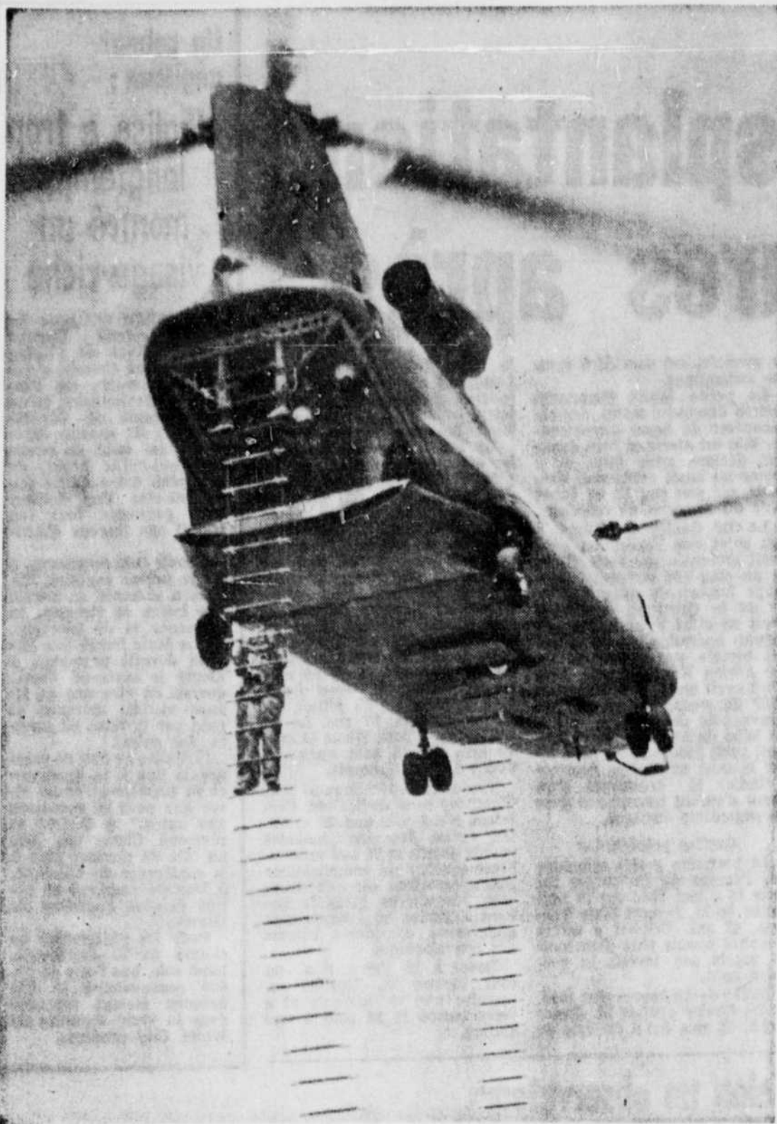
On a fait récemment la démonstration de ce nouvel appareil qui fera le transport des troupes dans la jungle et les marécages. Cet hélicoptère de type CH 47 Chinook a été présenté à Stockton en Californie. Vingt soldats peuvent monter à bord en l'espace de 4 minutes. Cela réduit de beaucoup la période de stabilité de l'hélicoptère de combat, au moment où les soldats montent à l'intérieur. L'appareil est actionné par un moteur de 43 HP.
