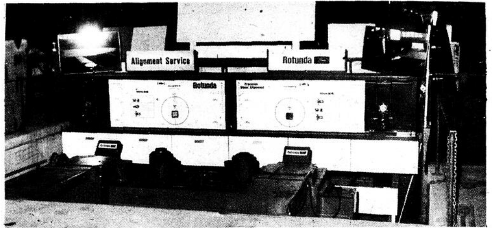
Machine à aligner pour poids lourds
