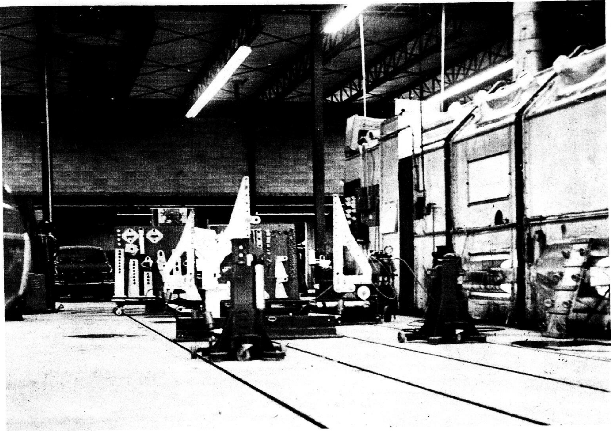
Redresseur de chassis Skanik pour poids lourds, importé de Suède
