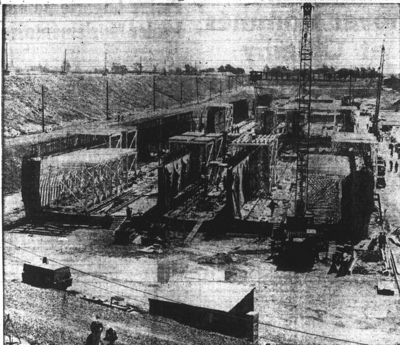
Le tunnel, du pont-tunnel Louis-Hyppolite-Lafontaine, commence à prendre forme dans l'énorme cale sèche qu'on a creusée à même le lit du St-Laurent. On voit bien les trois sections du tunnel, soit les deux tubes de circulation et le petit tube central pour la ventilation et l'entretien. Construit à ciel ouvert, le tunnel sera ensuite glissé dans le fleuve par sections longitudinales. Il y a un an que les travaux ont commencé sur ce chantier qu'a visité le ministre de la Voirie, M. Bernard Pinard, la semaine dernière. La construction du tunnel entre l'île de Montréal et l'île Charron et du pont entre celle-ci et la rive sud doit être complétée à la fin de l'automne 1966.
