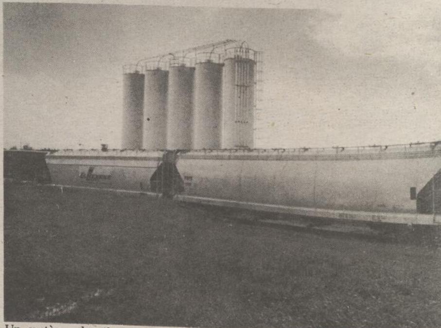
Un système de silos. Les résines qui formeront le plastique dont sont faits les contenants Tupperware sont emmagasinées dans des silos qu'on aperçoit de loin lorsqu'on arrive à Cowansville. De là, elles sont acheminées automatiquement aux machines.
