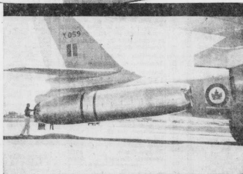
ESSAIS EN VOL DU NOUVEL IROQUOIS À MALTON Le moteur supersonique Iroquois est porté par un dispositif spécial fixé à l'arrière du B-47.
