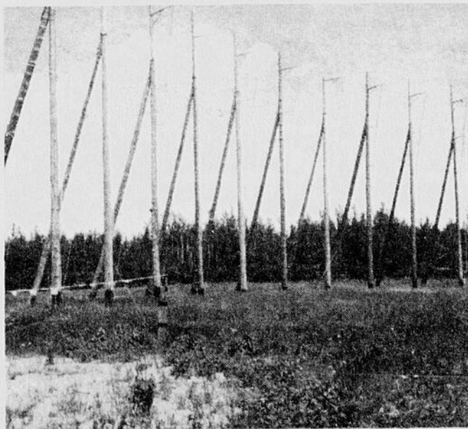
TOUR PARABOLIQUE de Dolbeau Télévision Inc. Cette Tour avec un écran de 50 pieds de haut par 150 pieds de long capte les ondes des deux postes
