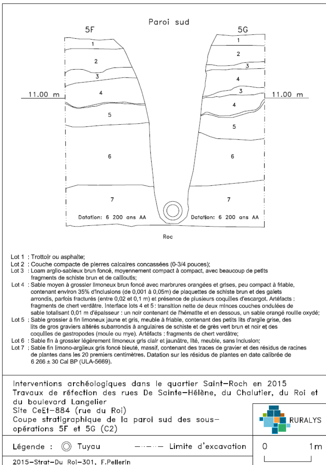
Figure 43. Coupe stratigraphique de la paroi sud des sous-opérations 5F et 5G (C2)
