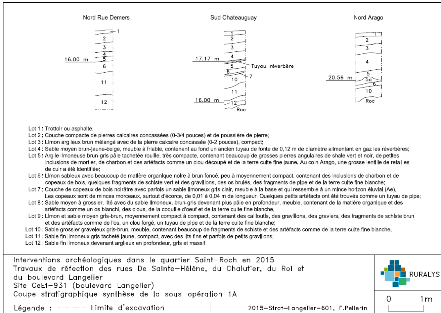
Figure 31. Coupe stratigraphique synthèse de la sous-opération 1A du site CeEt-931
