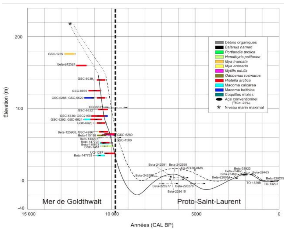
Figure 4. Tableau représentant les fluctuations du niveau marin entre 12 000 ans et 1 000 ans AA dans la région de Québec (Lamarche 2011 : 87)
