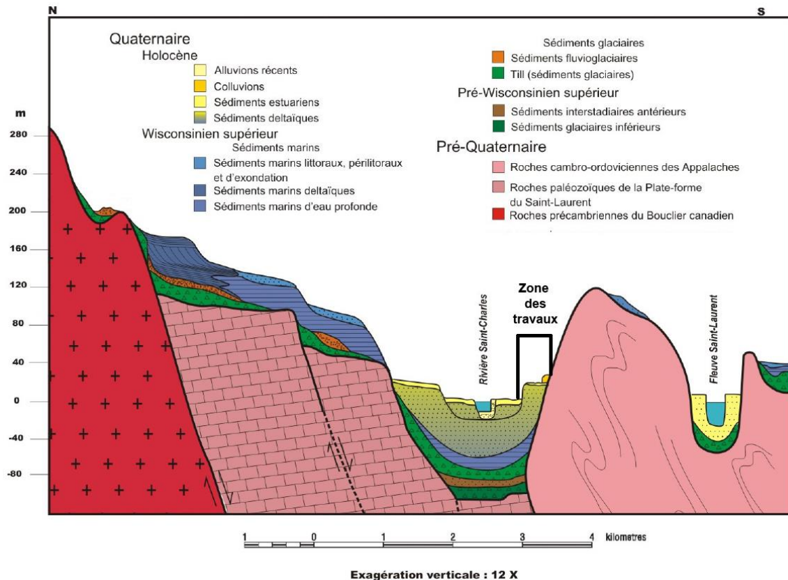
Figure 2. Coupe géologique de la région de Québec dans laquelle est positionnée la zone générale des travaux (Carte tirée de Lamarche 2011 : 96)
