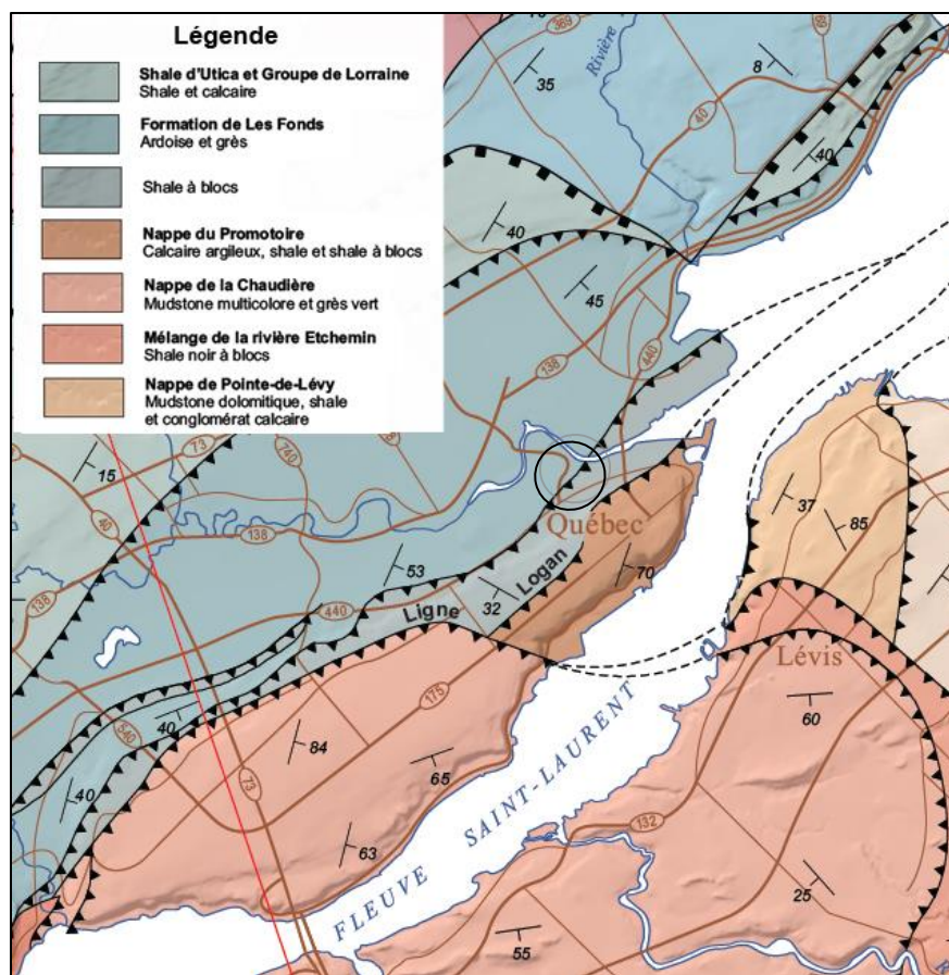
Figure 3. Détail de la carte géologique simplifiée de la région de Québec. Le cercle noir localise de manière générale le quartier Saint-Roch (Castonguay et Nadeau 2012)
