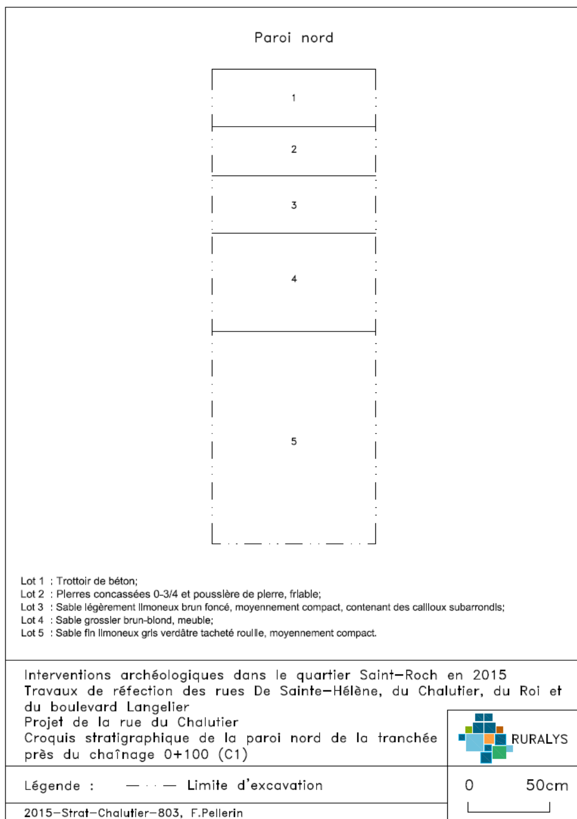
Figure 26. Croquis stratigraphique de la paroi nord de la tranchée près du chaînage 0+100 (C1)
