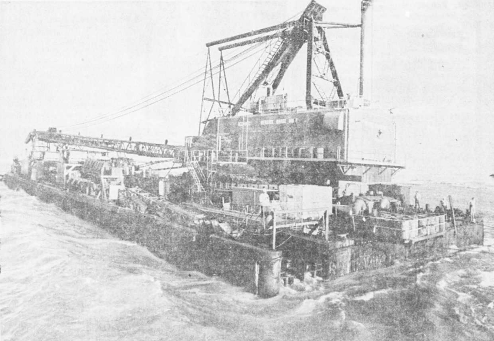
Ce chaland à derrick est le plus impressionnant du genre utilisé présentement au large des côtes égyptiennes, sur les champs pétroliers de Morgan. Le chaland comporte un équipage de 135 hommes qui dorment sous les ponts dans un confort air climatisé et la grue peut soulever jusqu'à 250 tonnes de matériel lors de la pose de pipeline sous-marin.
