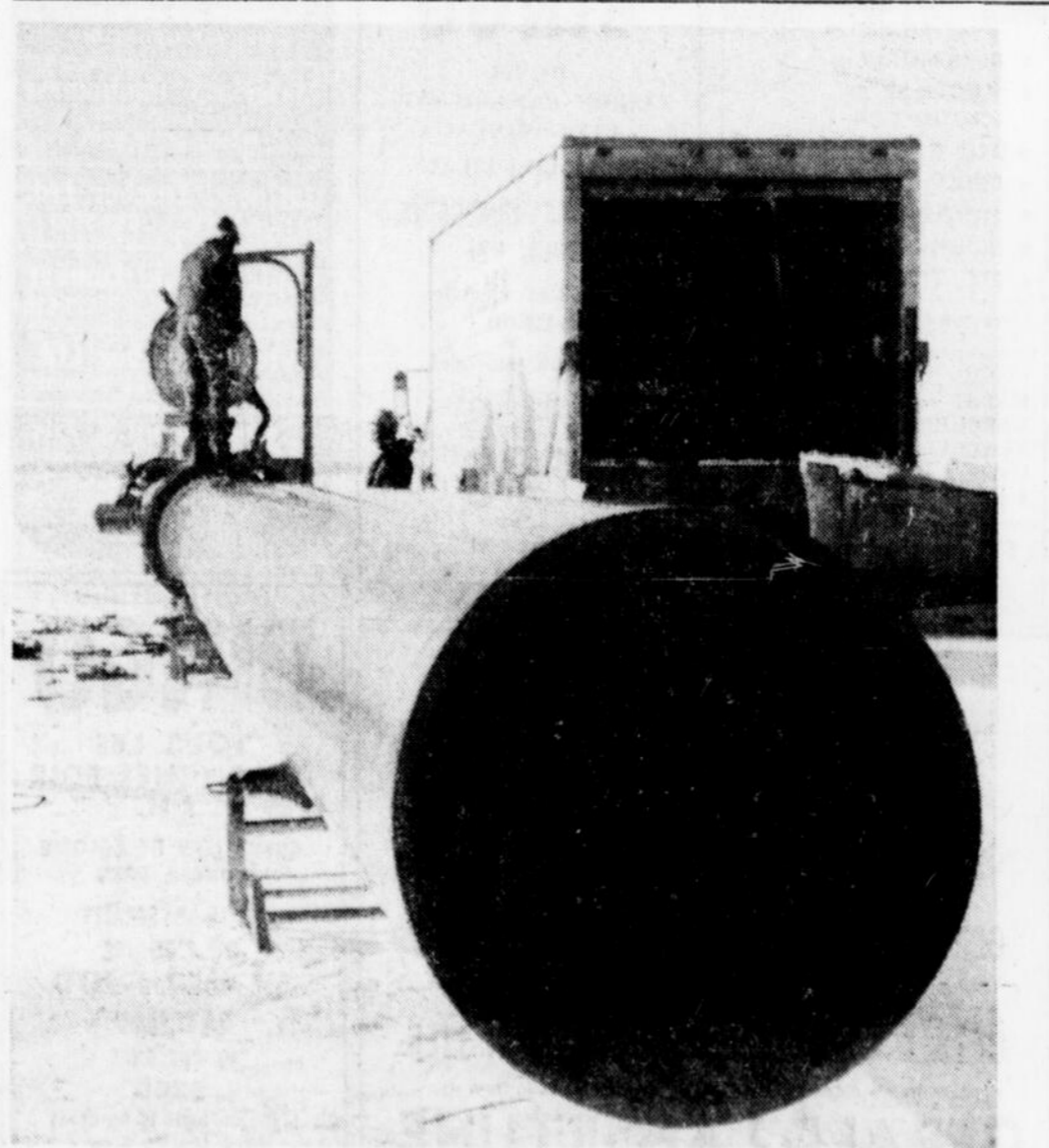
BOUCHE DE CANON? — Les travaux d'installation des tuyaux de l'usine de filtration d'Aylmer vont bon train. Les ouvriers de Thom Construction sont en train de joindre cette section de 28 pouces de diamètre à la conduite d'amenée, qui aura plus de 2,500 pieds de longueur entre l'usine et le lac.
