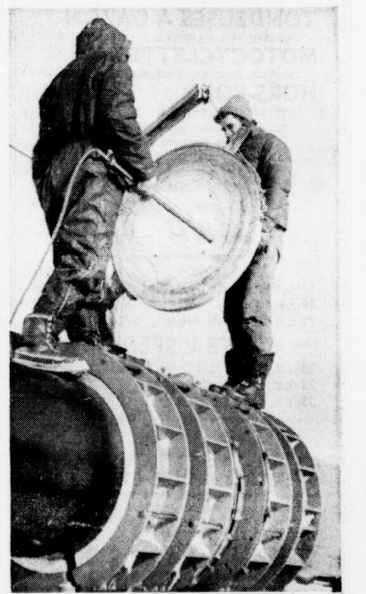
METHODE DE SOUDURE — Pour relier les sections du tuyau d'alimentation de la nouvelle usine de filtration d'Aylmer, les ouvriers doivent chauffer une plaque pour fondre les deux bouts de tuyau et les souder. Selon M. Germain Pigeon, gérant du bureau de Thom Construction, à Hull, c'est la première fois qu'on tente une telle expérience avec ce genre de tuyau, dont l'extrémité doit reposer à trente pieds sous l'eau. On devra couper la glace du lac Des Chênes pour l'immerger.
