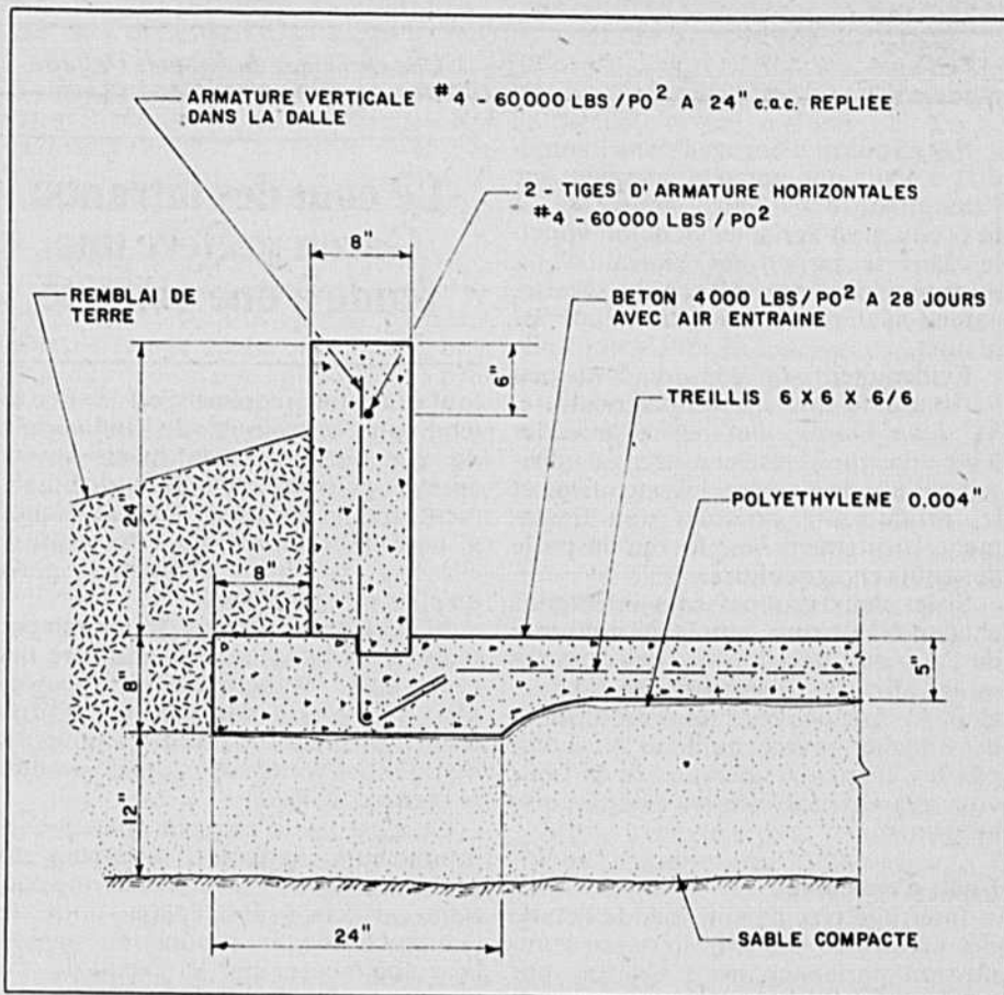
Coupe indiquant les dimensions de la dalle, des murs, l'armature requise et le remblai nécessaire pour une plate-forme pour montée de nettoyeur d'étable.
