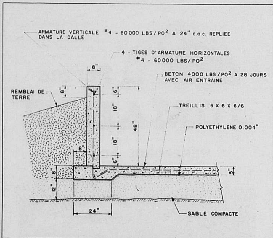
Coupe indiquant les dimensions de la dalle, des murets, l'armature requise et le remblai nécessaire pour une plate-forme pour évacuateur souterrain.
