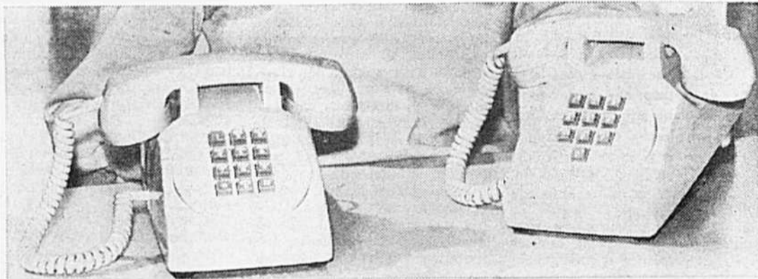
A droite, c'est l'appareil standard à dix poussoirs, actuellement en usage au Canada. A gauche, c'est le téléphone de demain: ses 2 touches supplémentaires, appelées préfixe et suffixe, donneront accès à des services révolutionnaires. Il est présentement fabriqué par Northern Electric.
