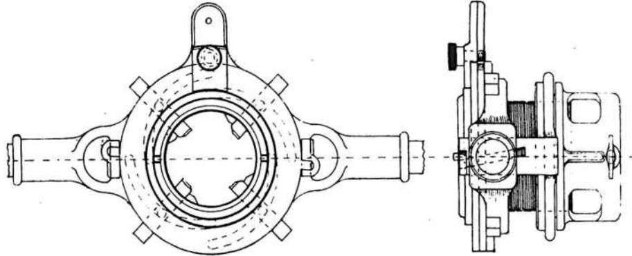
Filière montrant les comes et les peignes à fileter ajustables
