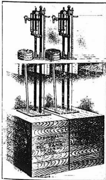
Gravure No. 35. Double Appareil de cave pour Deux Sortes d'Huile.
